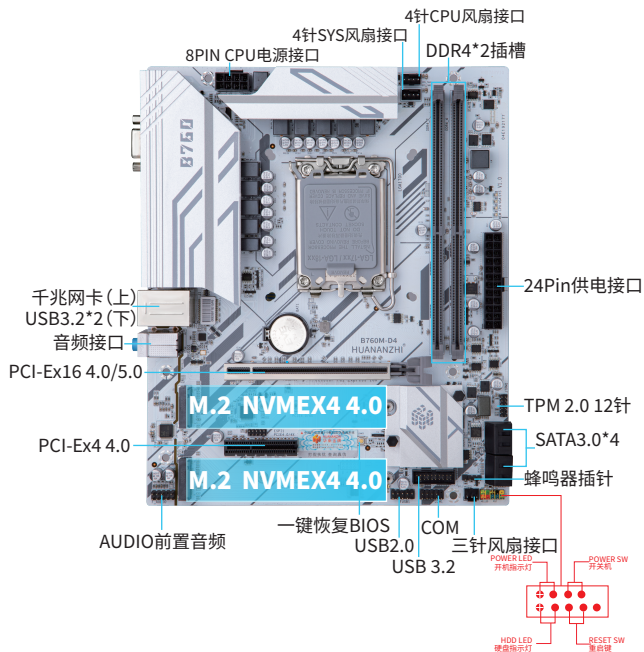
1-1 B760M-D4主板图解
