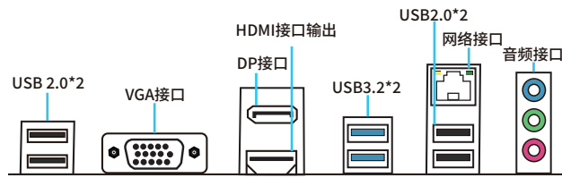
1-2 整体后置I/O面板展示
