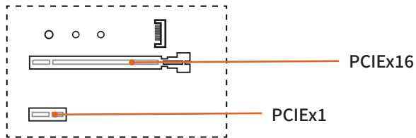
图2-4 PCI扩展插槽
