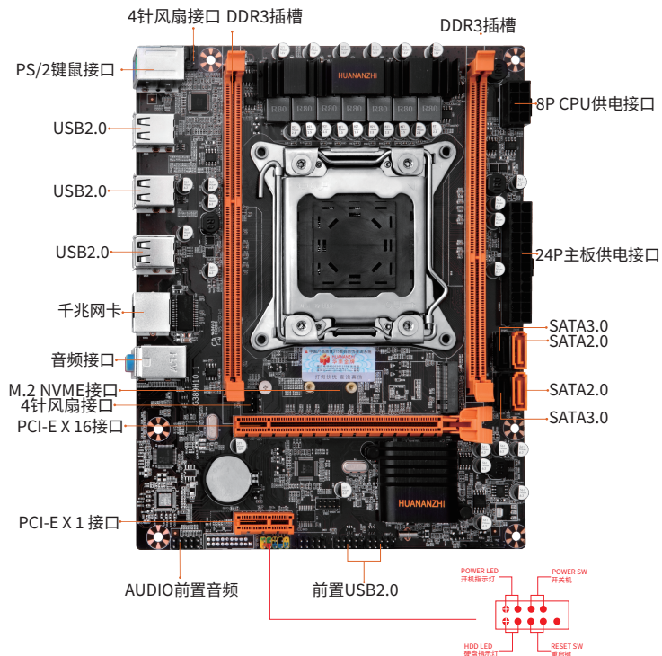
图1-1 X79-4M V2.0主板图解
