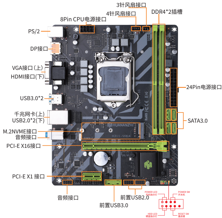
图1-1 H311-VHD4主板图解
