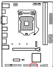
图2-3 USB扩充接口
