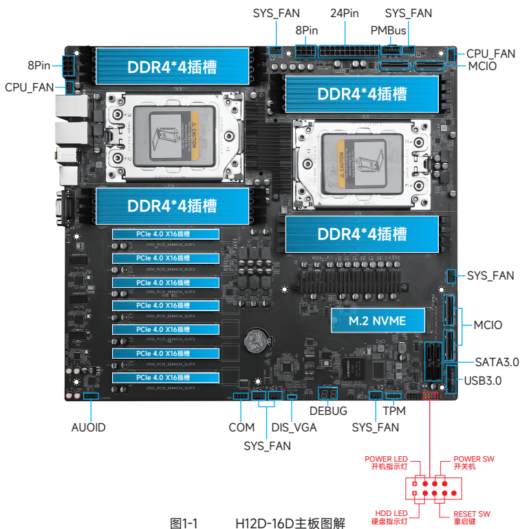
图1-1 H12D-16D主板图解
