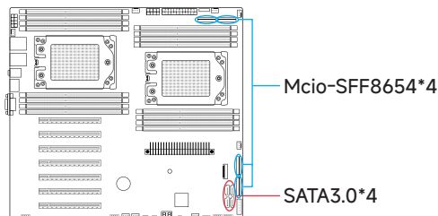
图2 -10 SATA接口
