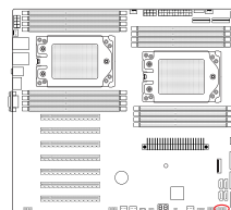
图2-3 PCI扩展插槽
