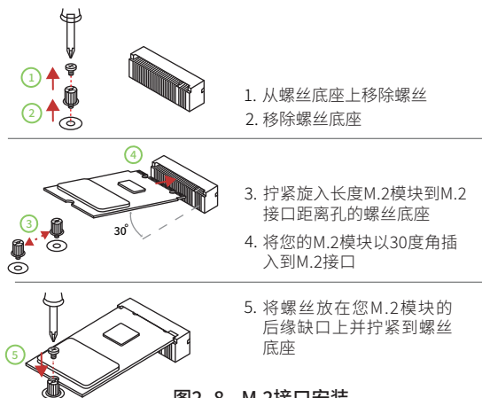
图2-8 M.2接口安装
