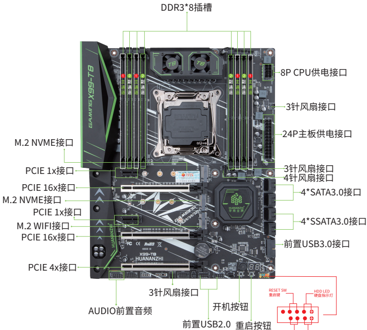
图1-1 X99-T8主板图解
