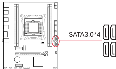
图2 -10 SATA接口
