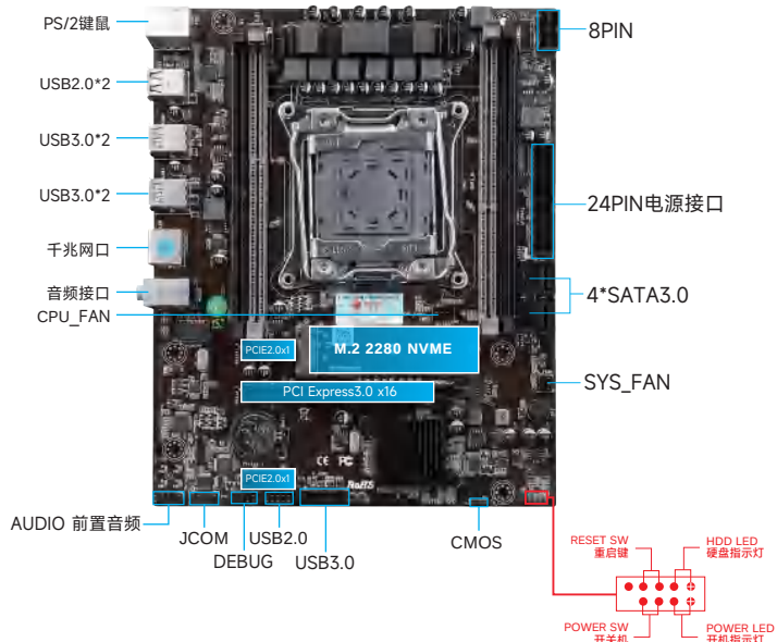
图1-1 X99-MTF主板图解
